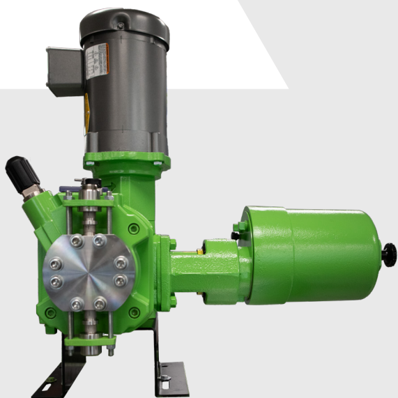
PulsaPro 680 - 880 - 7120
