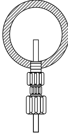
Resim 6 Fışkırtma noktalı ventilin borulara bağlantısı
