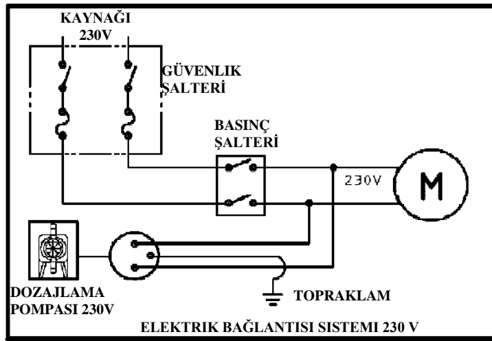
Resim 8 Kuyu pompasının tipik elektrik bağlantısı
